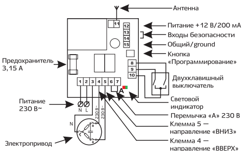
Рис. 1 — Подключение Radio 8113 IP65
