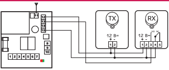
Рис. 6 — Подключение ИК-барьера
