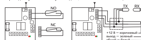
Рис. 4 — Подключение геркона
