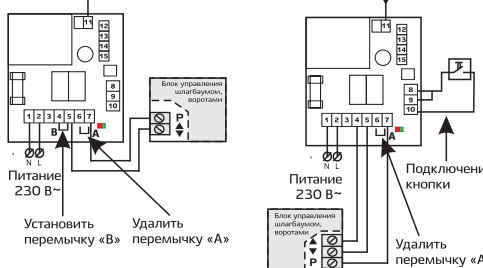
Рис. 2 — Подключение к пошаговому входу
